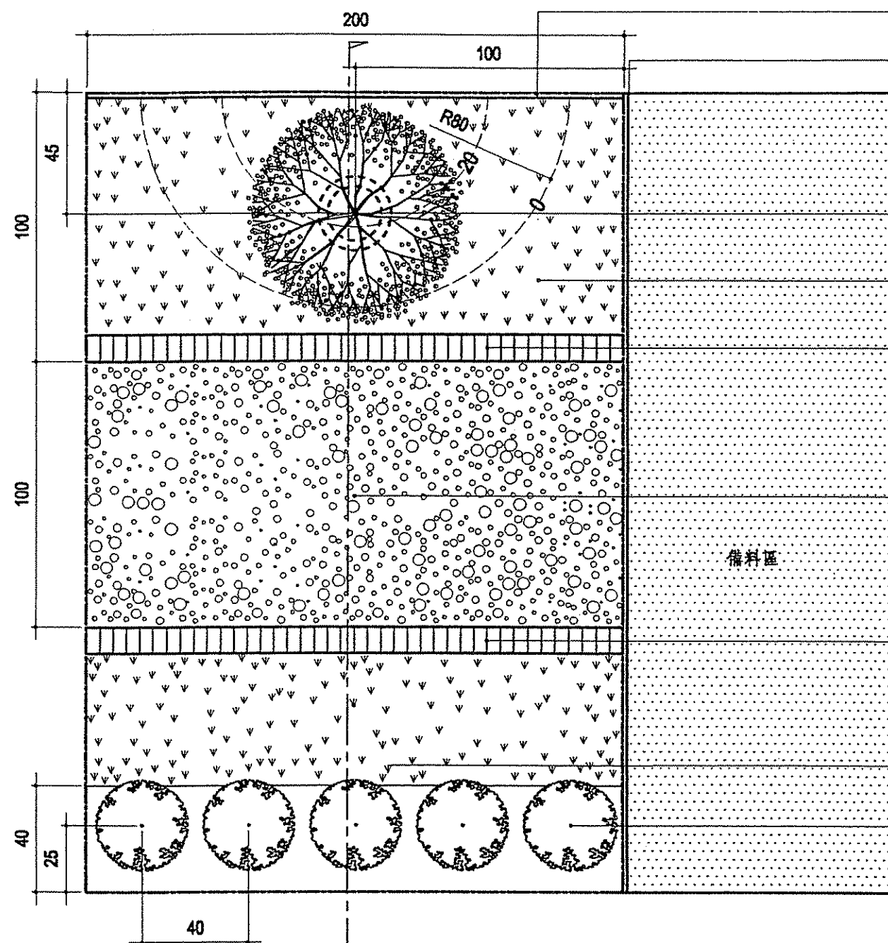
平面圖 S=1/20
