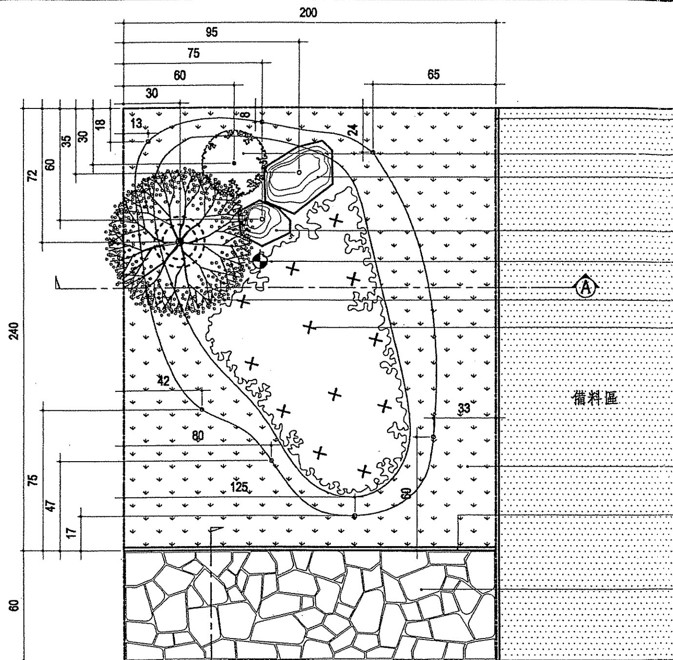
平面圖 S=1/20
