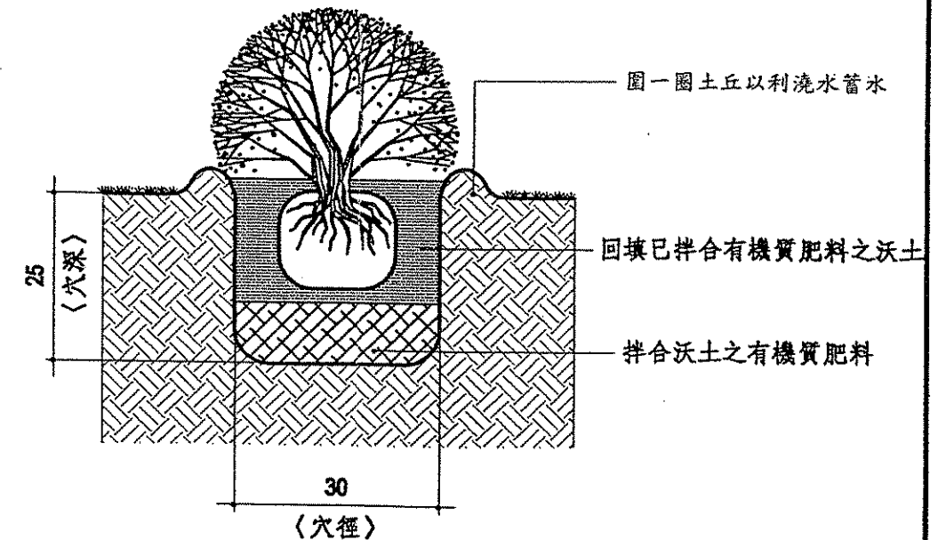
灌木種植剖面示意圖 S=1/10
