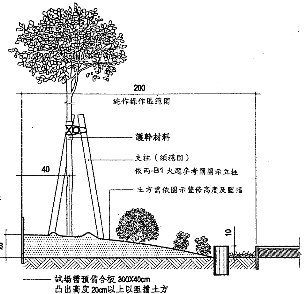
剖面圖 A S=1/20
