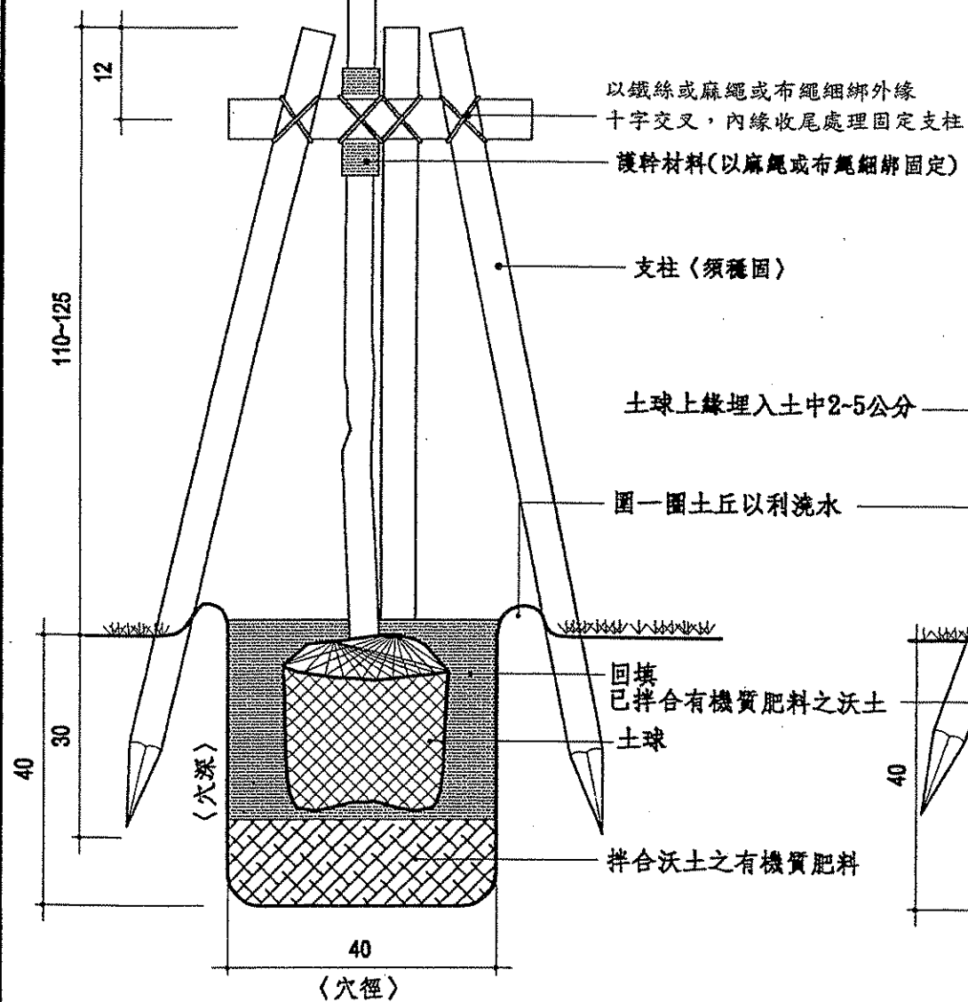
喬木栽植剖面示意圖 S=1/10
