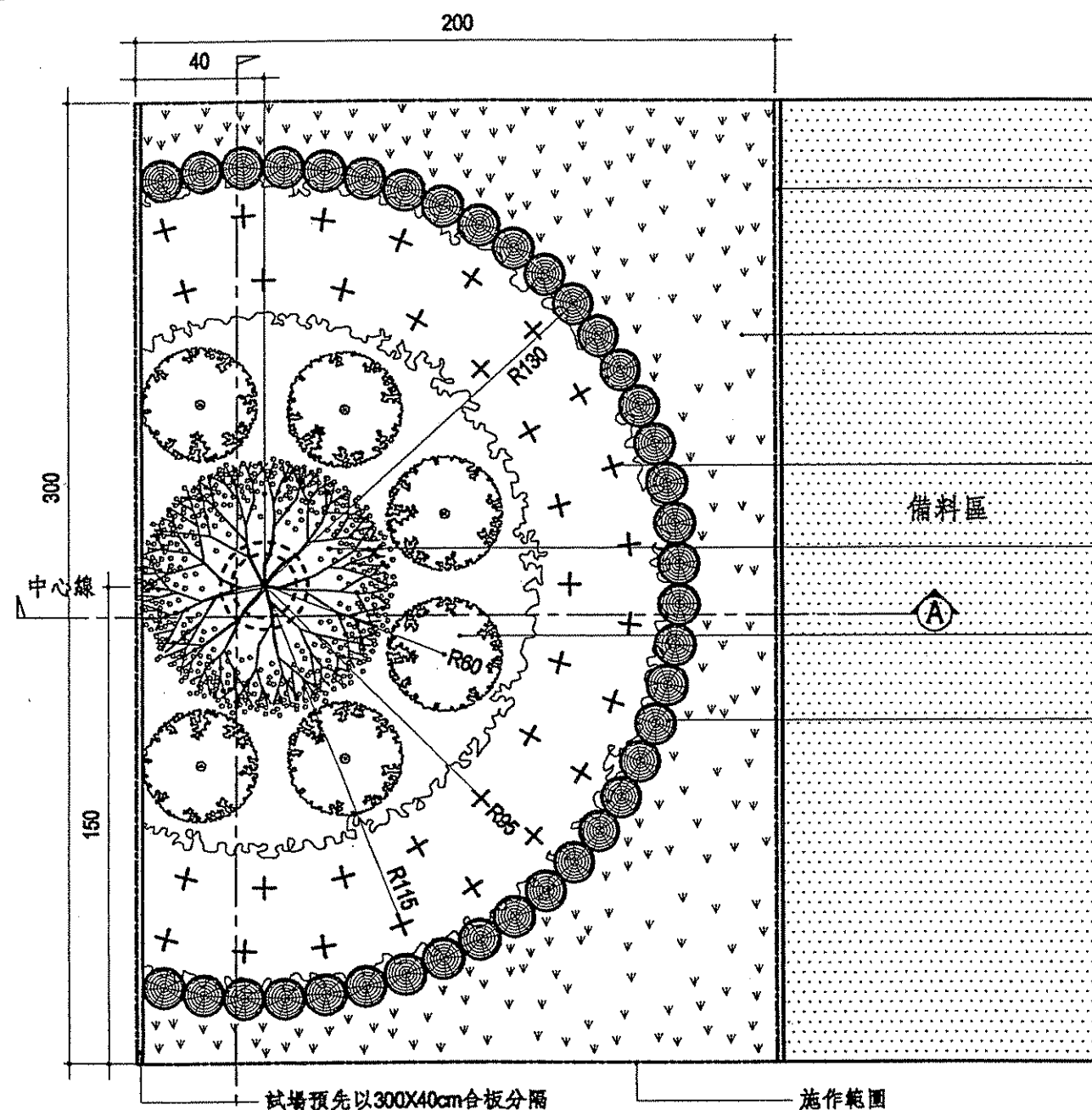
平面圖 S=1/20
