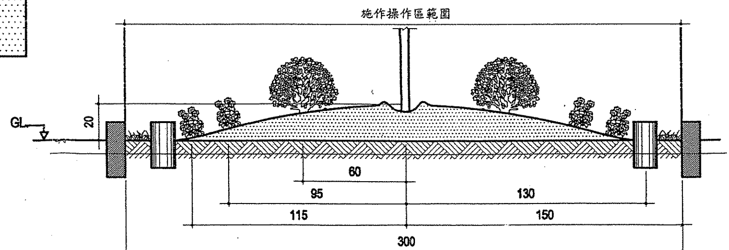
剖面圖 B S=1/20
